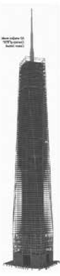
◆（圖二）世貿一號大樓的結構透視圖底層外牆厚達10米，大樓中心直通屋頂的脊椎一米厚之高強度混凝土防爆耐撞的承重牆
